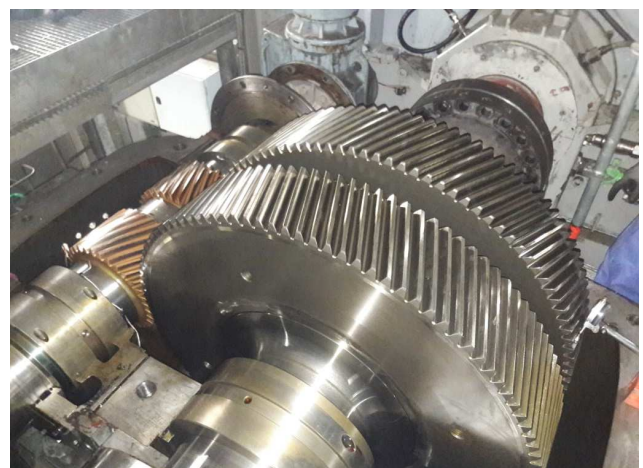
Ouverture et contrôle du réducteur du groupe turbo alternateur pendant révision mineure
